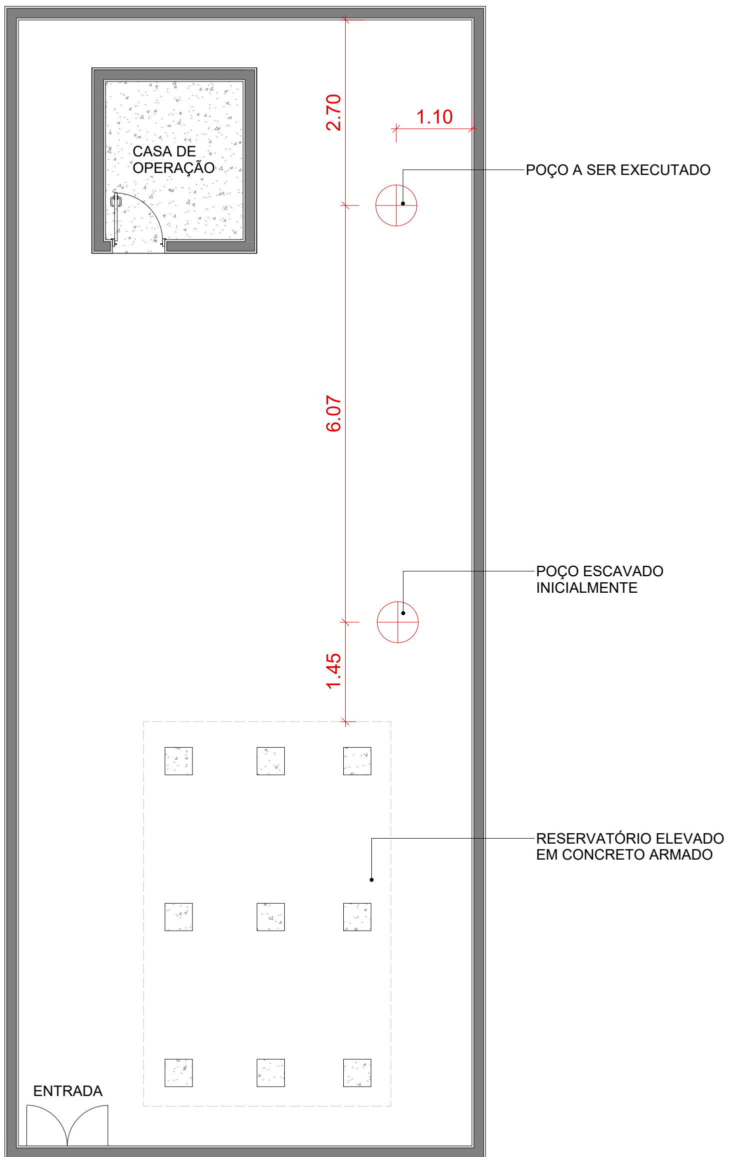
PLANTA DE LOCAÇÃO 1 : 50
